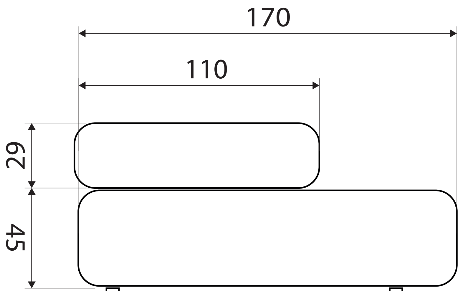
WIDOK BOK
