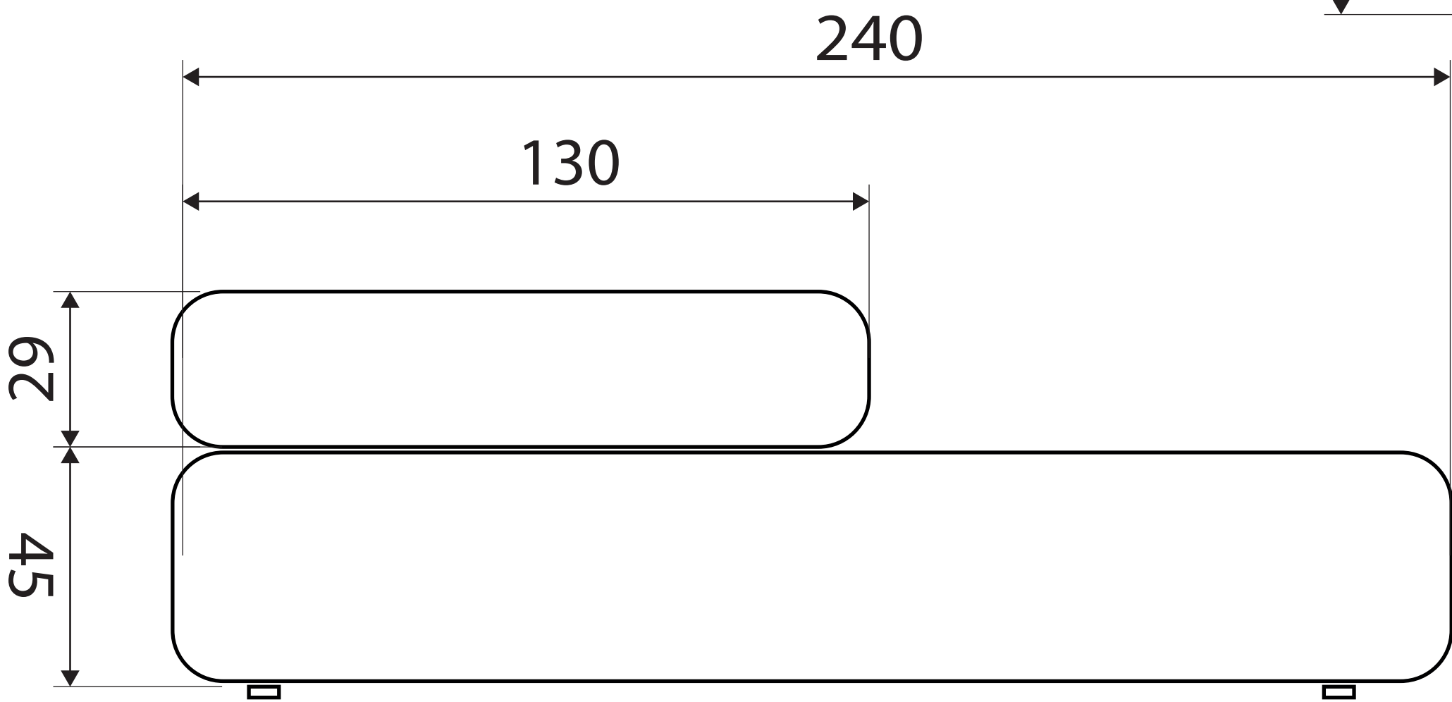
WIDOK FRONT
