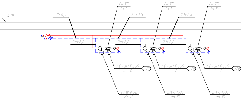
Instalacja CO dla Pomieszczenia Księgarni
